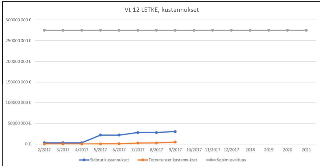
Kuva 2. Hankkeen kustannukset 9/2017
