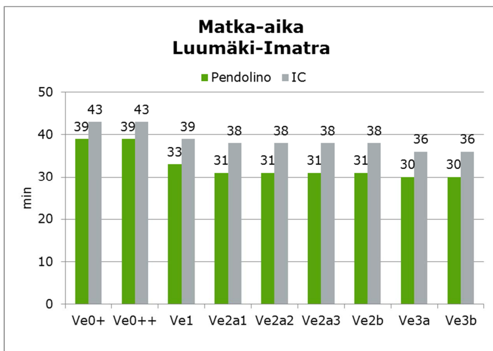
Kuva 20. Henkilöliikenteen matka-aika Luumäki–Imatra.
