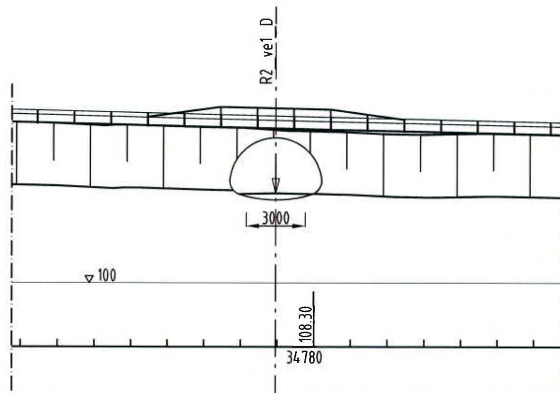
S27 PITUUSLEIKKAUS, 1:200
