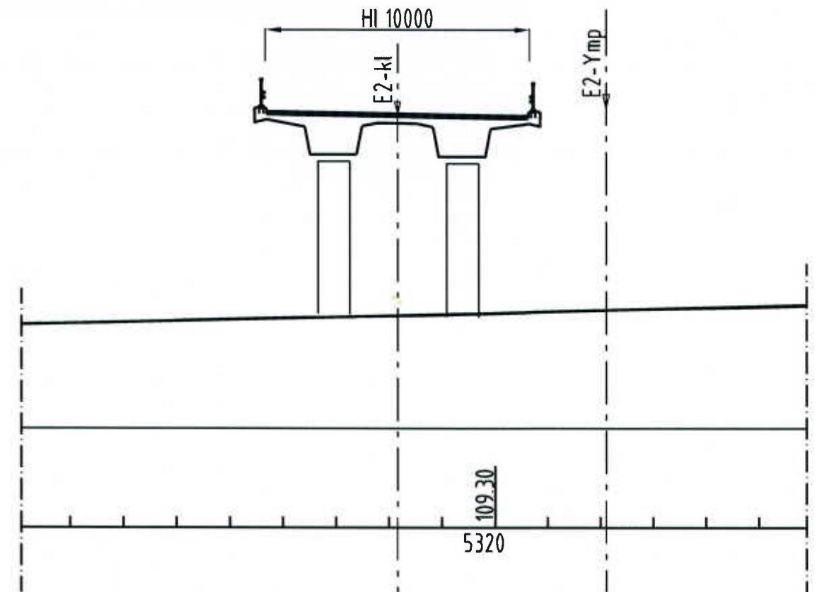
S8 A POIKKILEIKKAUS, 1:200
