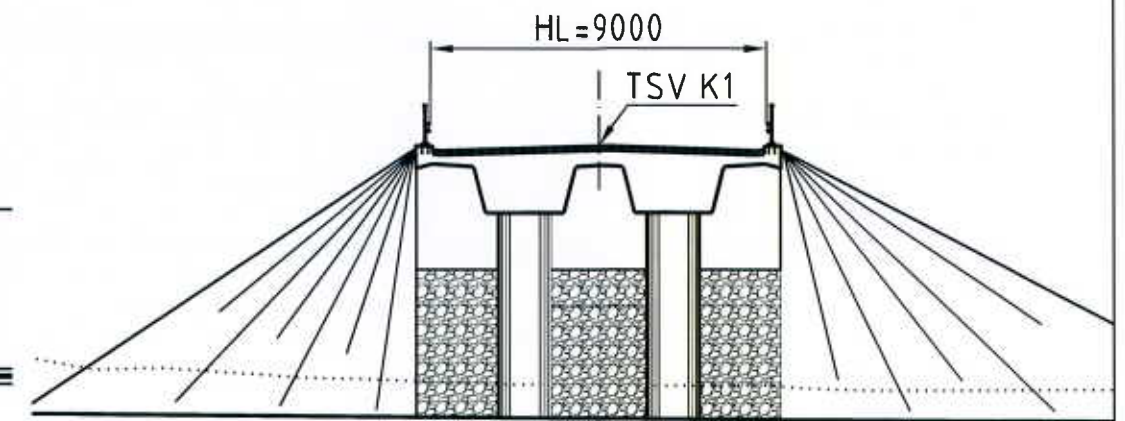
S2 POIKKILEIKKAUS B-B, 1:200
