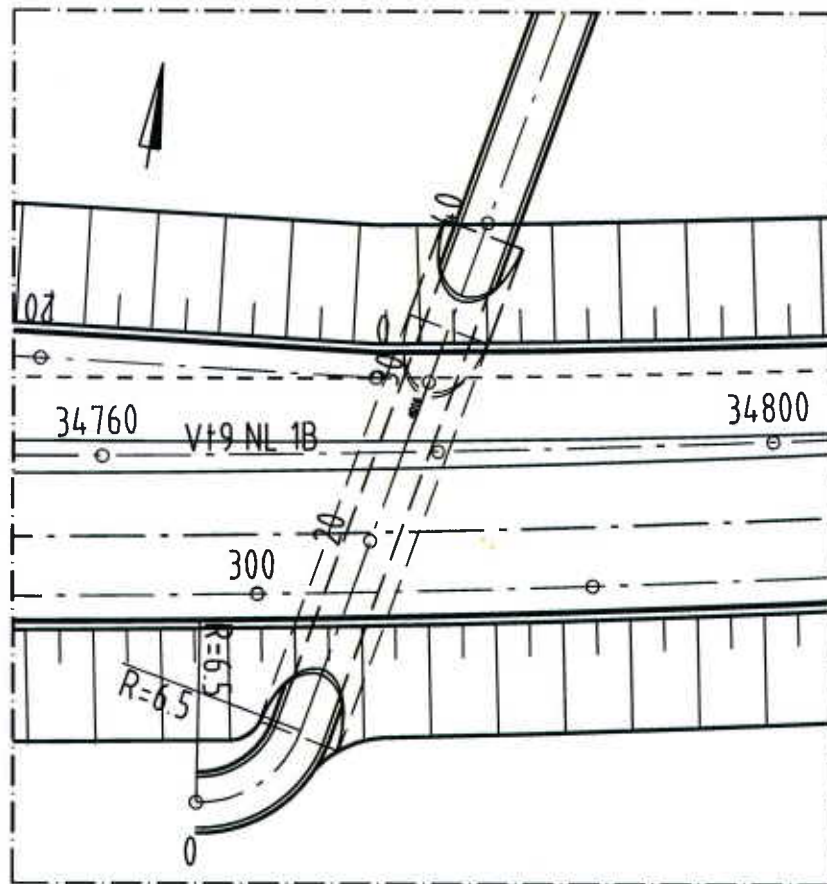
S 27 TASOPIIRUSTUS, 1:500
