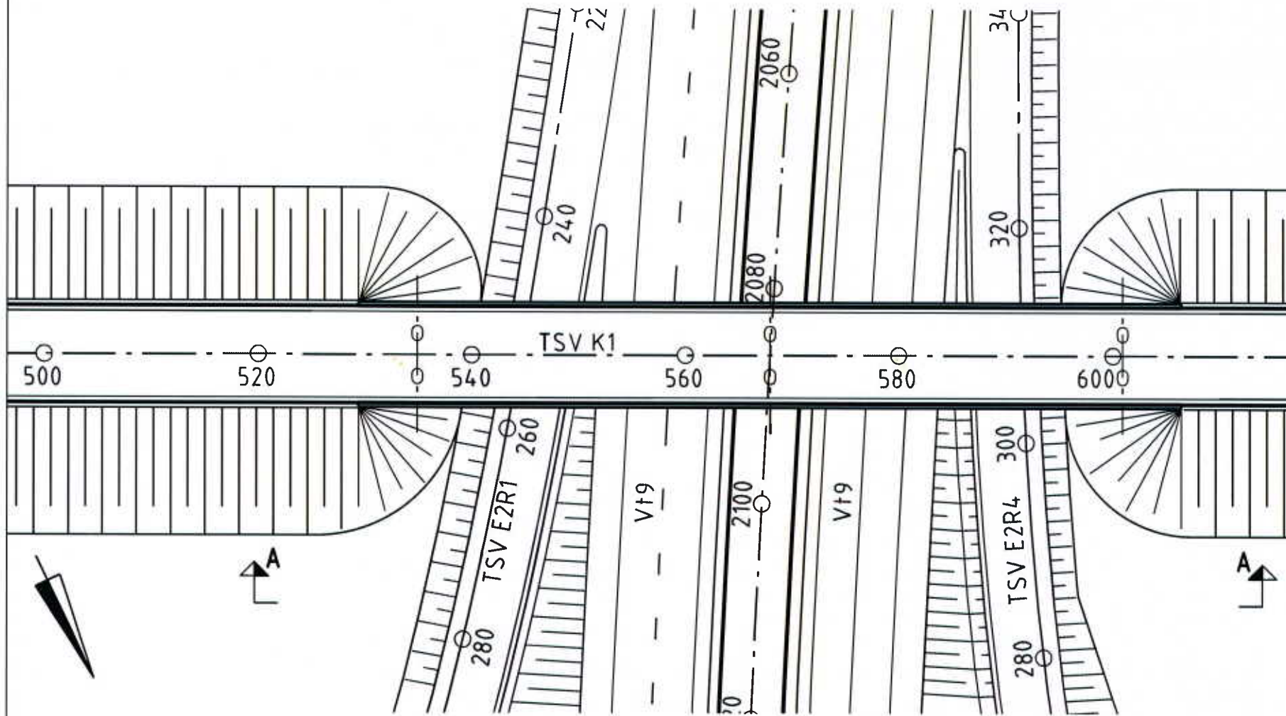
S2 TASOPIIRUSTUS, 1:500
