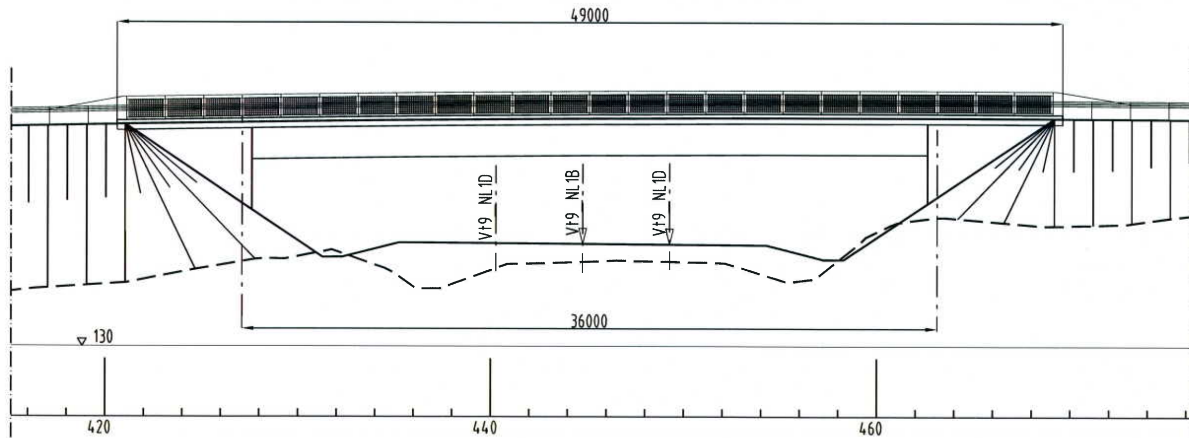
S13 PITUUSLEIKKAUS, 1:200
