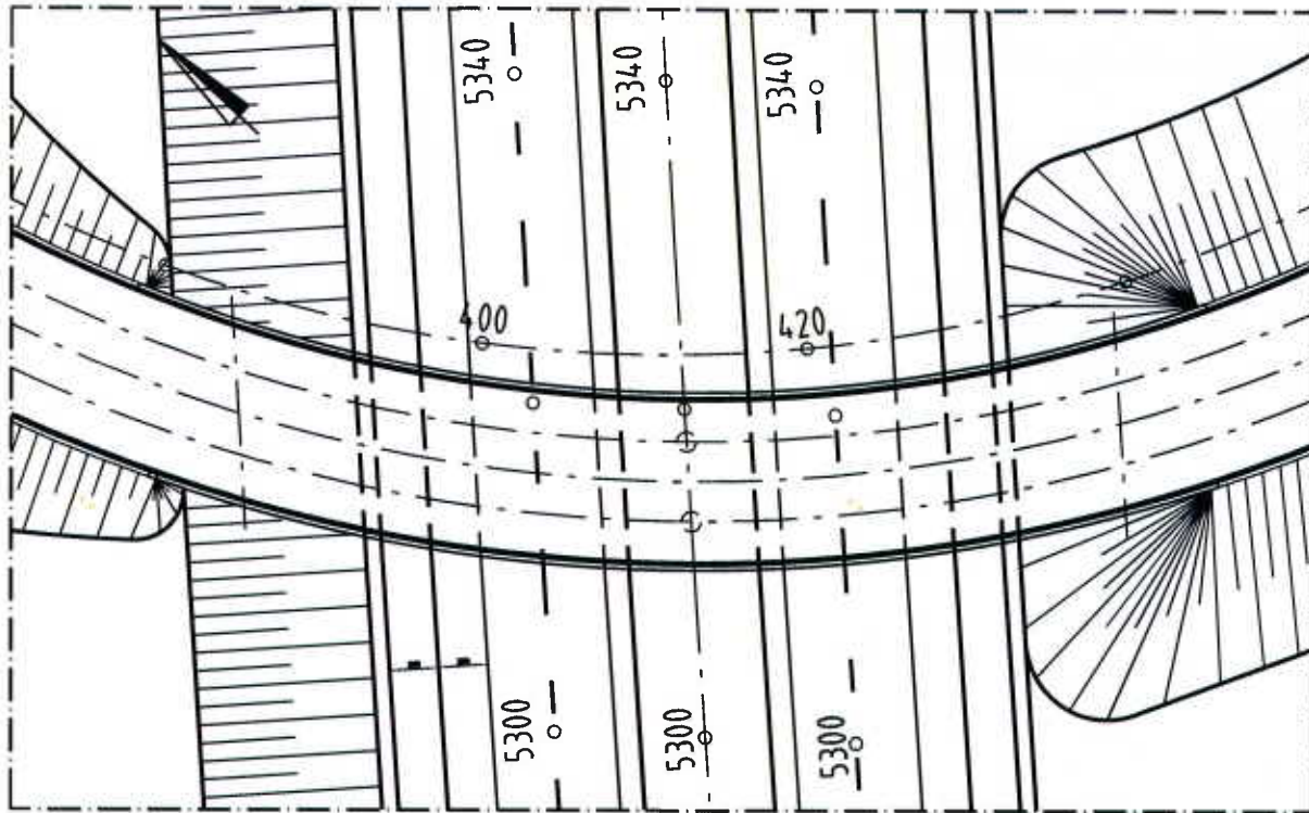
S8 A TASOPIIRUSTUS, 1:500
