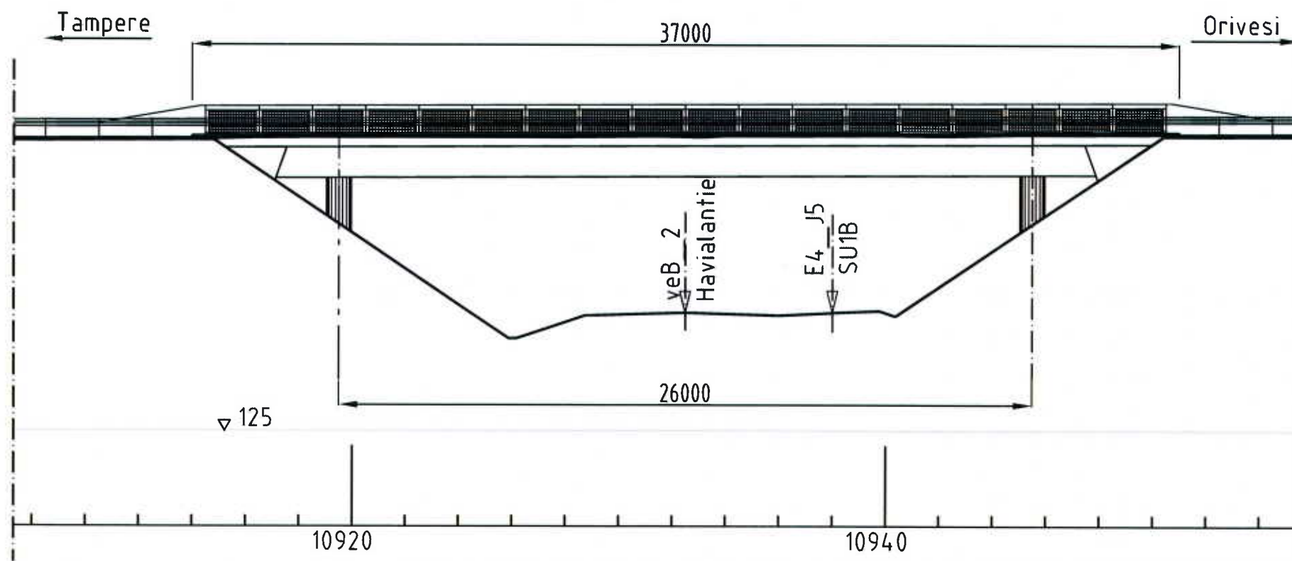
S14 PITUUSLEIKKAUS A-A, 1:200
