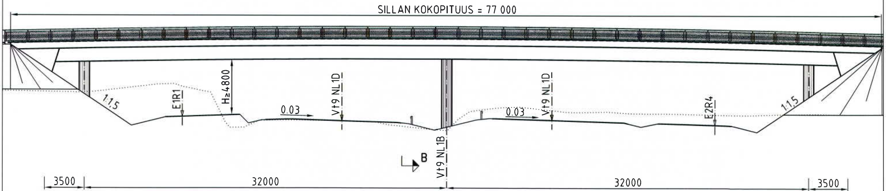
S2 PITUUSLEIKKAUS A-A, 1:200
