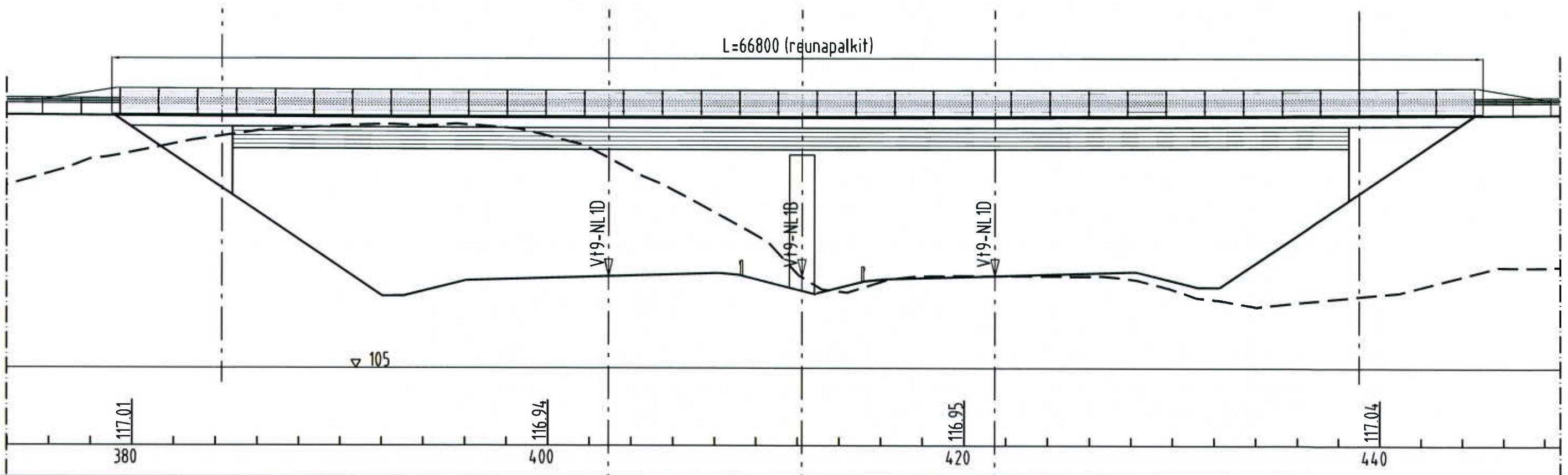
S8 A PITUUSLEIKKAUS, 1:200
