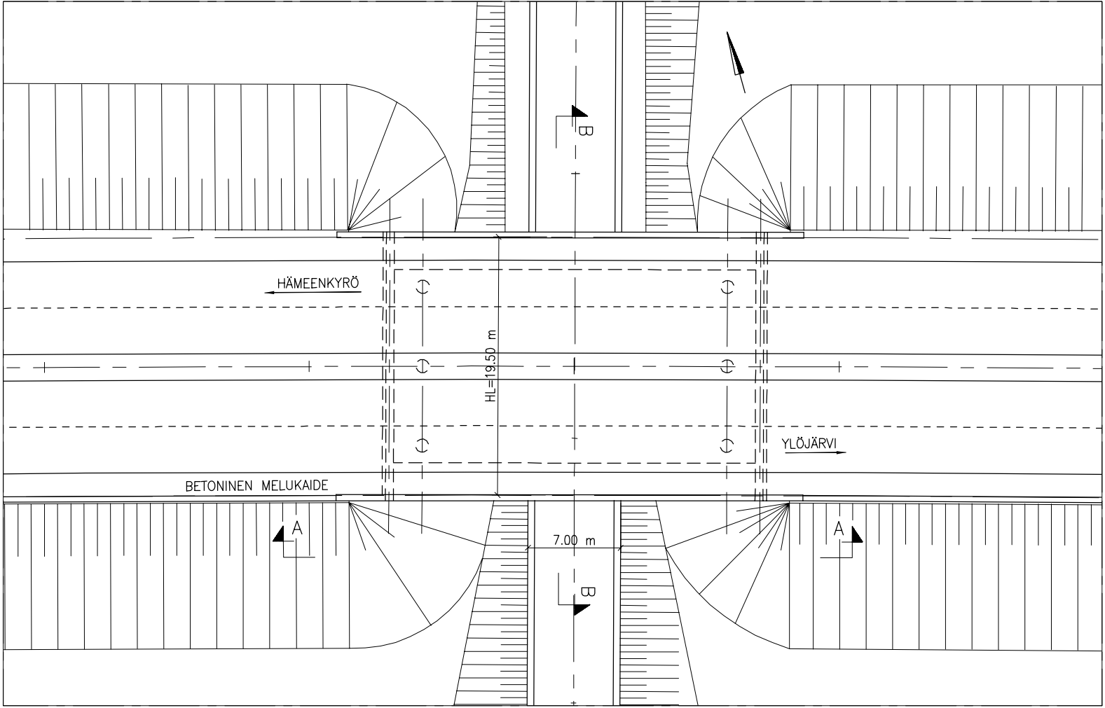
TASOKUVA 1:400
