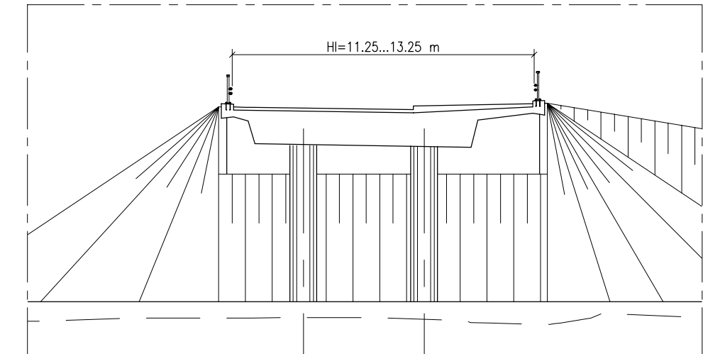
B - B 1:200
