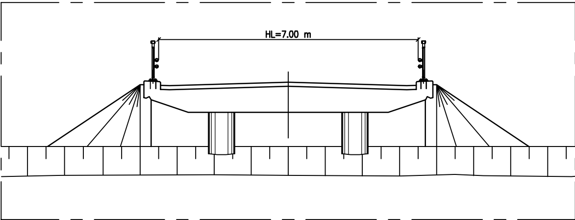
B - B 1:100
