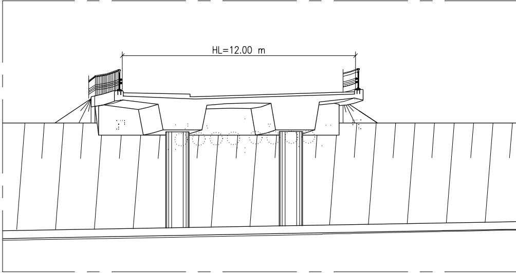
B - B 1:200
