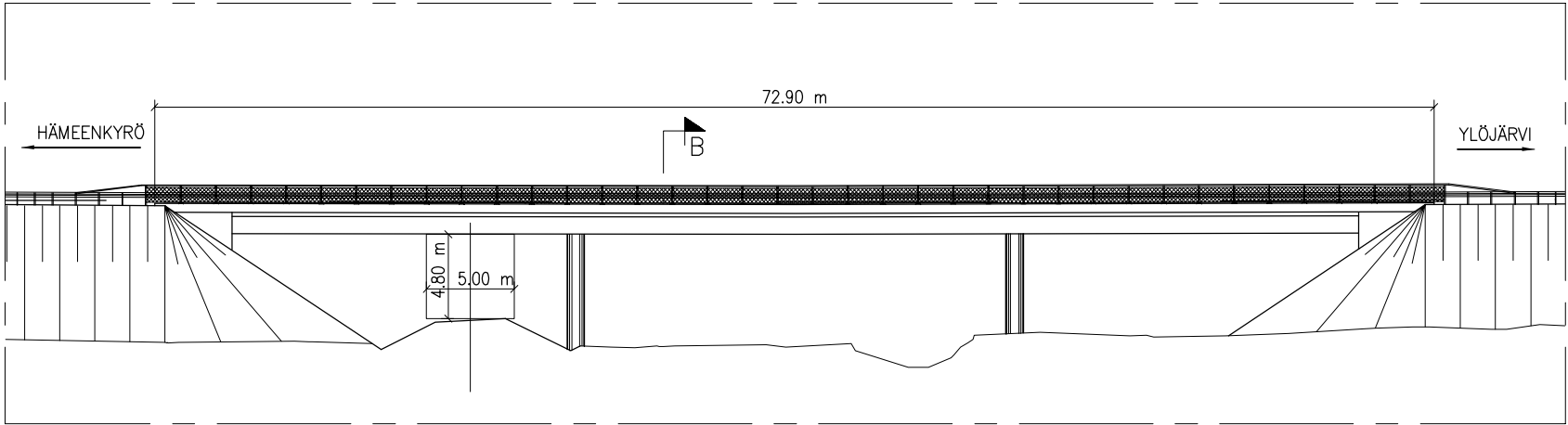
A - A 1:400
