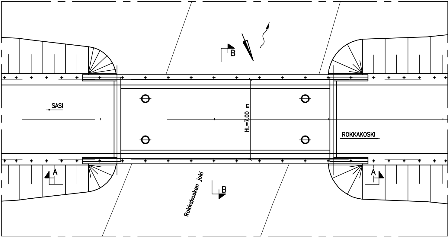
TASOKUVA 1:200
