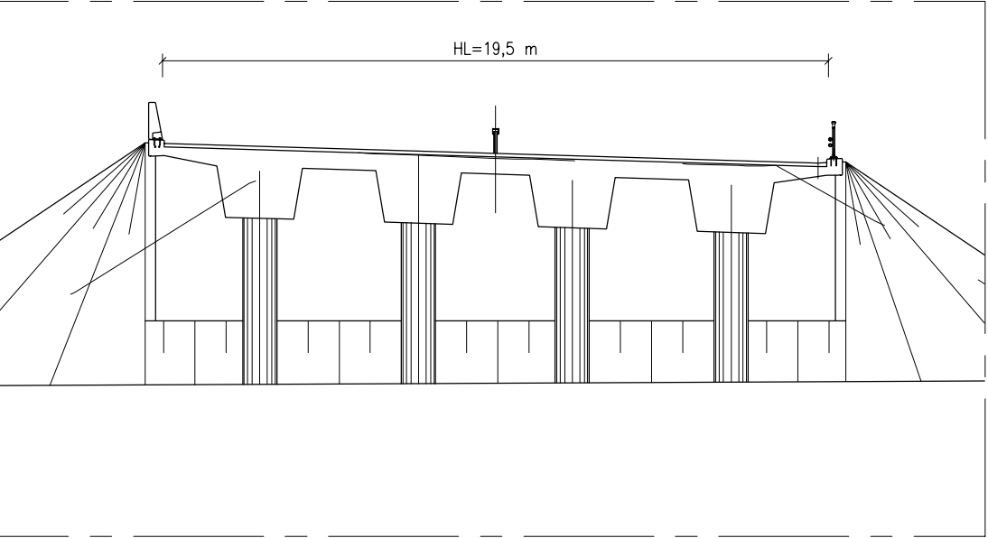
B - B 1:200
