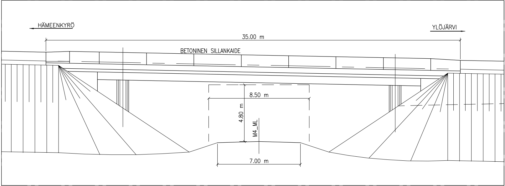
A - A 1:200
