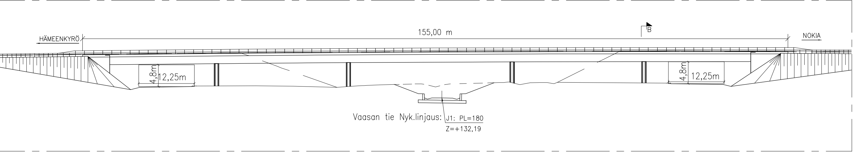
A - A 1:500
