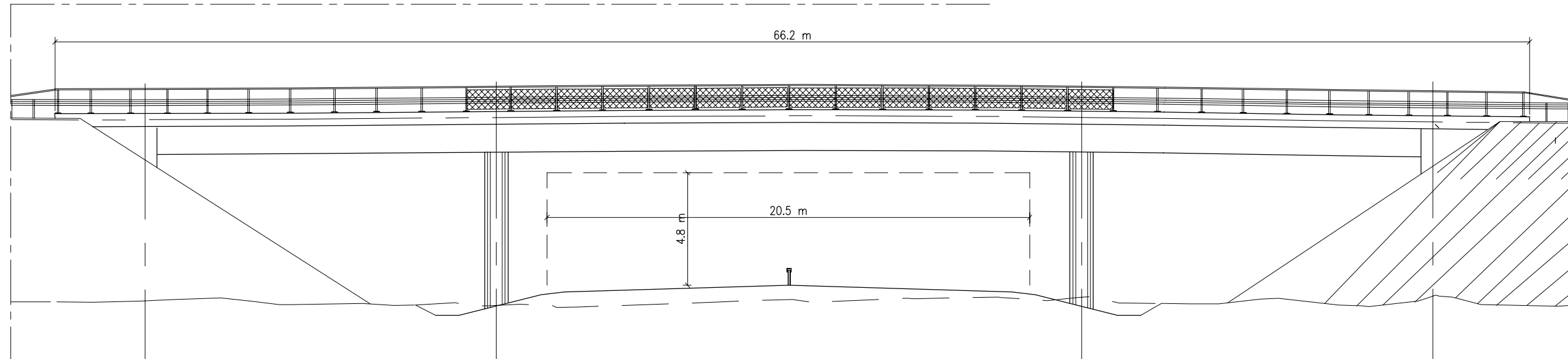
A - A 1:200
