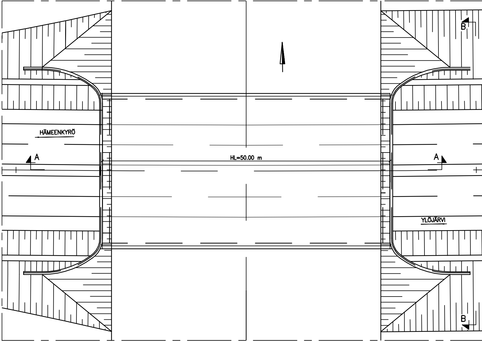
TASOKUVA 1:400
