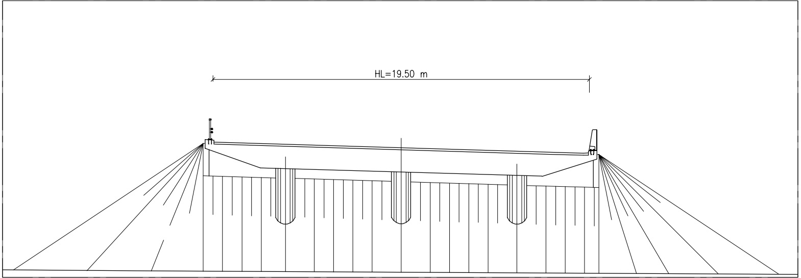
B - B 1:200
