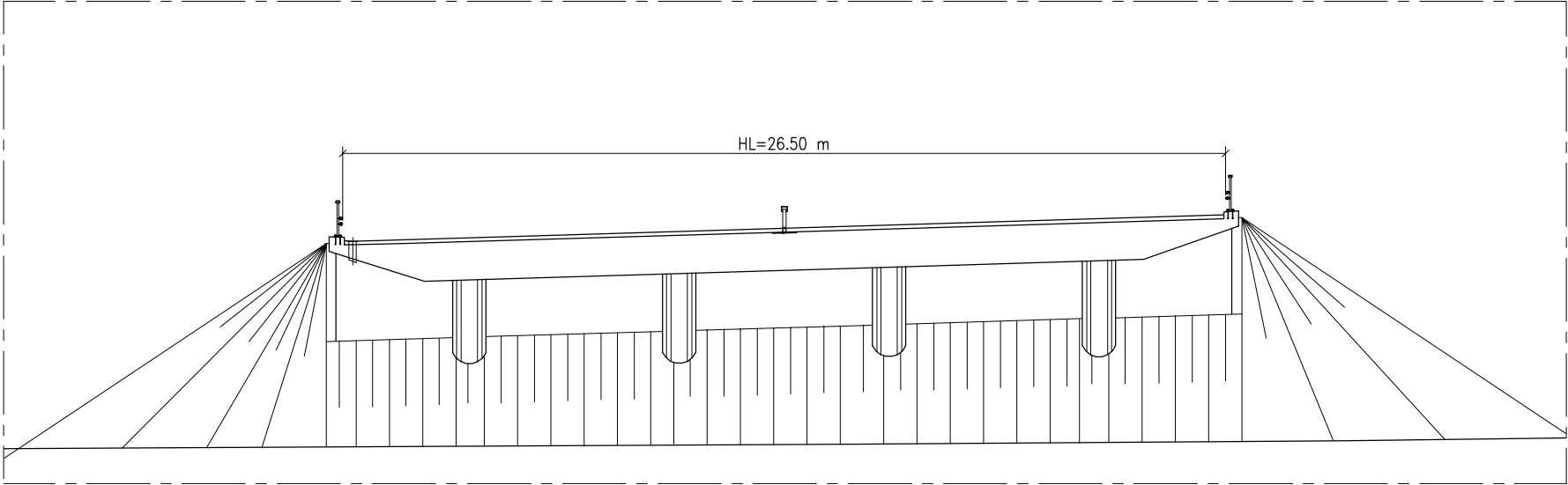
B - B 1:200
