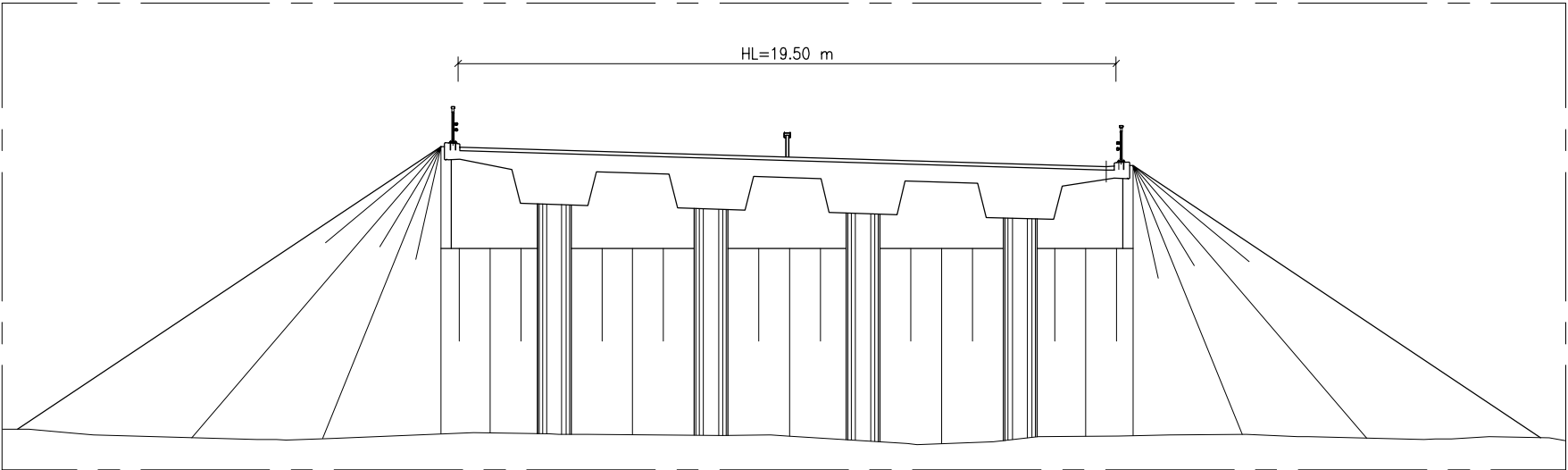
B - B 1:200
