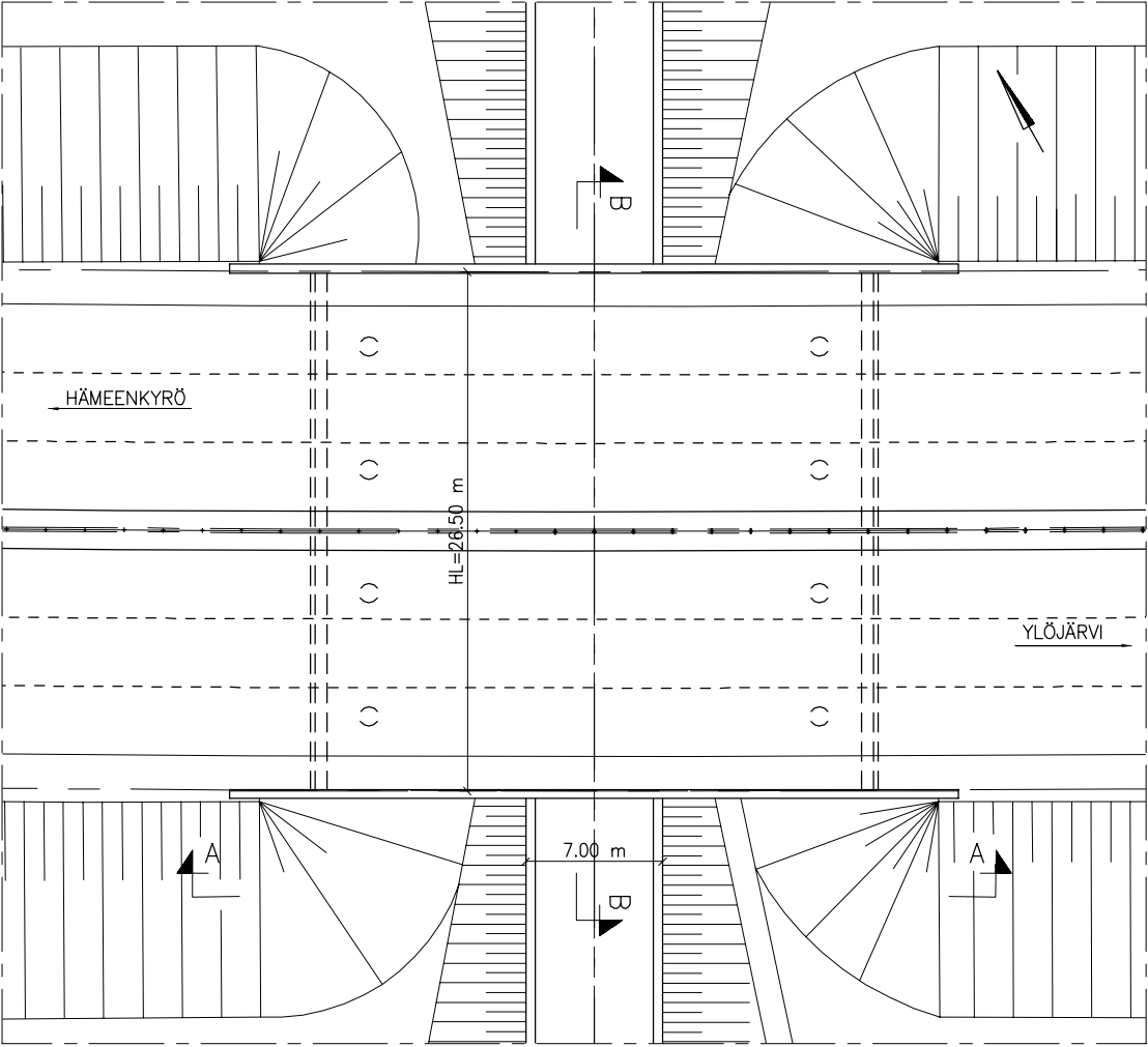
TASOKUVA 1:400
