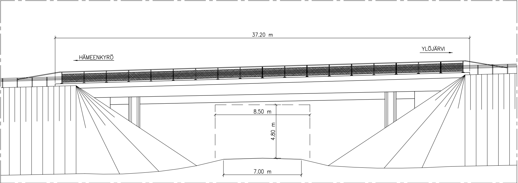
A - A 1:200
