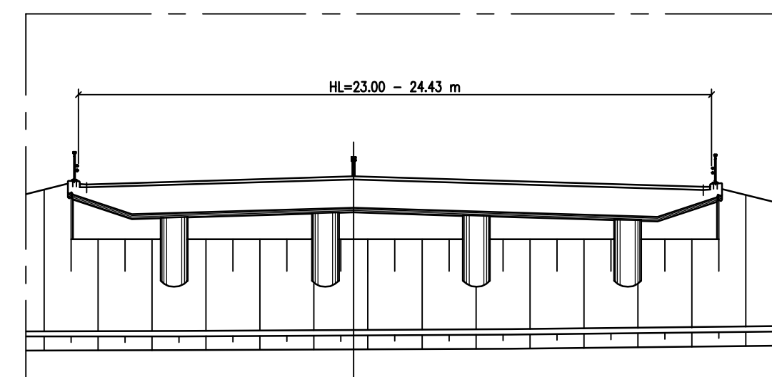
B - B 1:200
