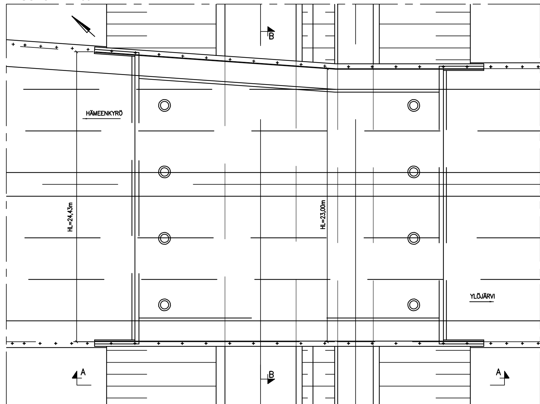
TASOKUVA 1:200
