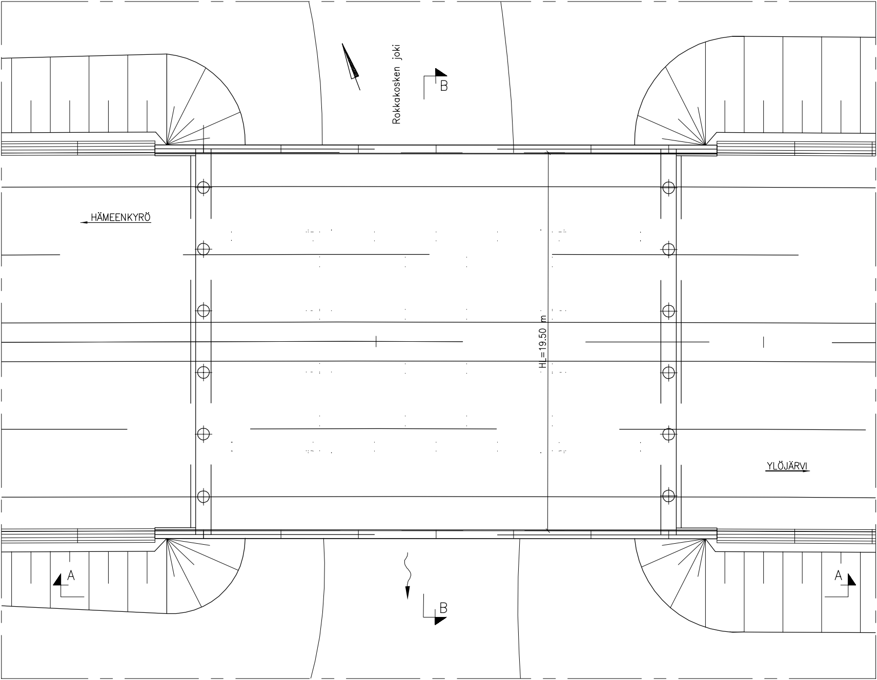
TASOKUVA 1:200
