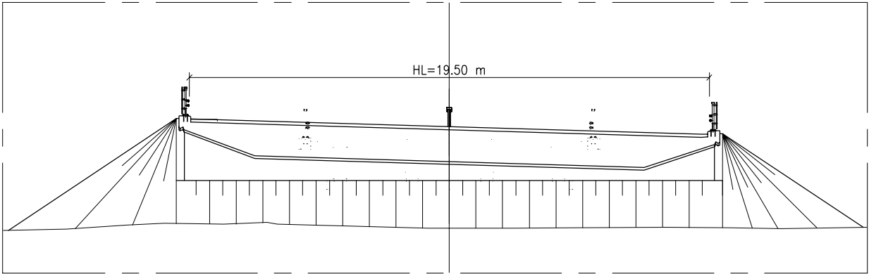
B - B 1:200
