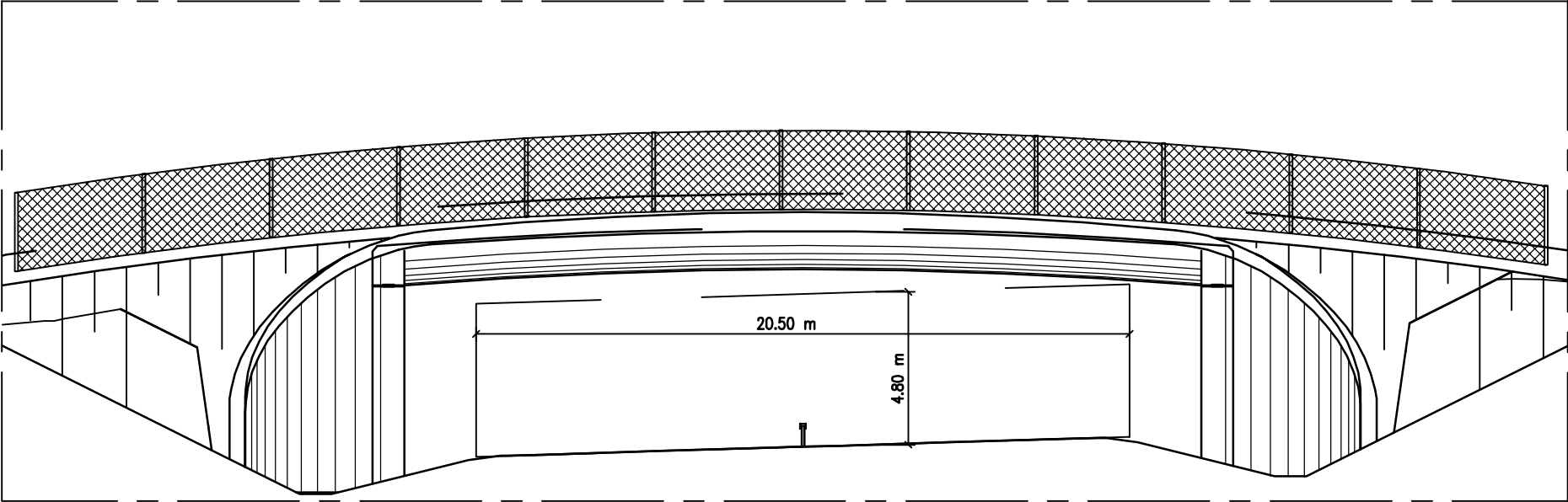
B - B 1:200
