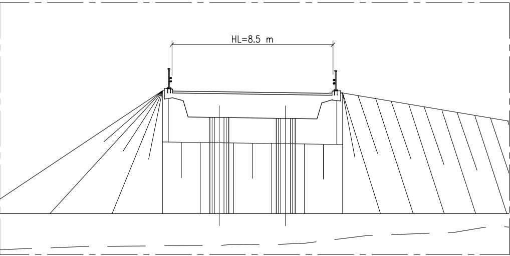
B - B 1:200
