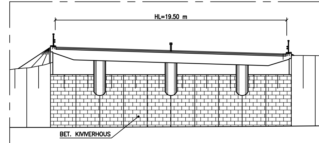
B - B 1:200
