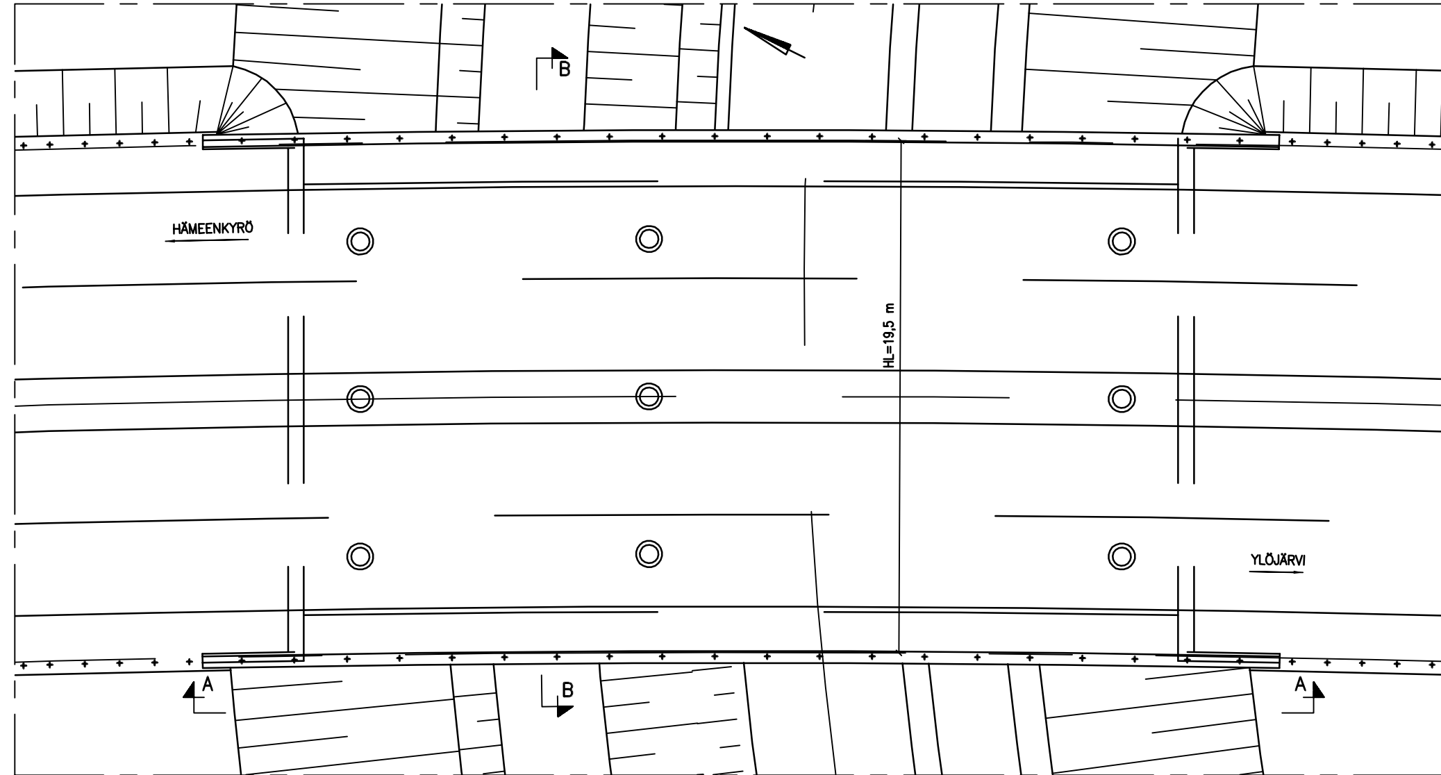
TASOKUVA 1:200
