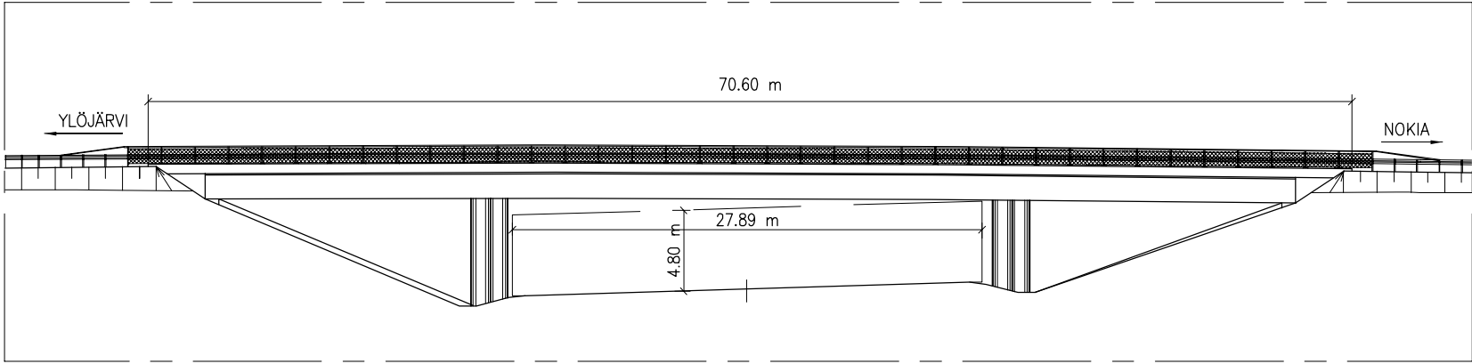
A - A 1:400
