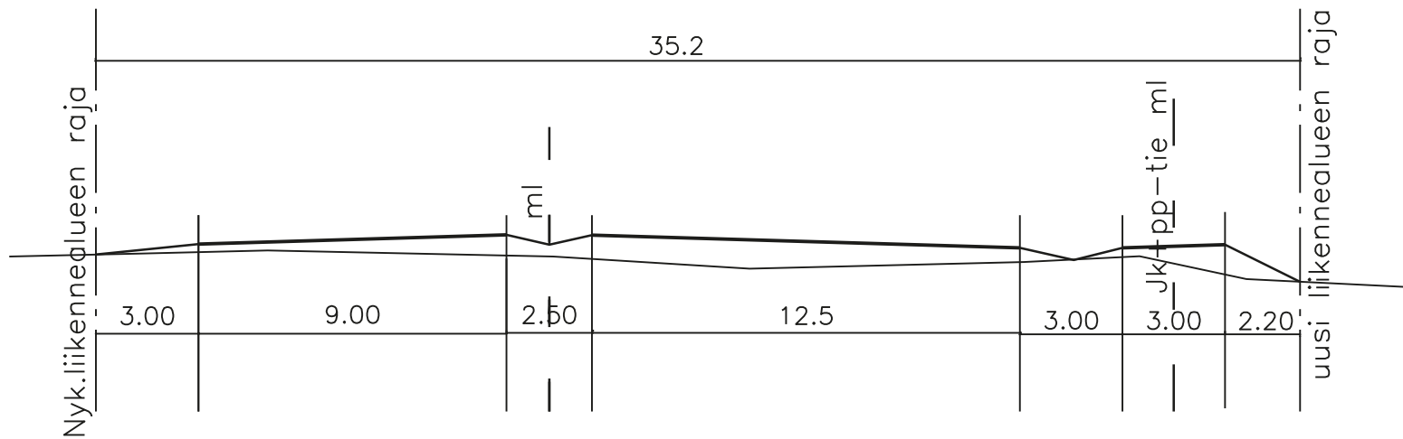
Laukaantien 2-ajoratainen poikkileikkaus ja oikealle kääntymiskaista
