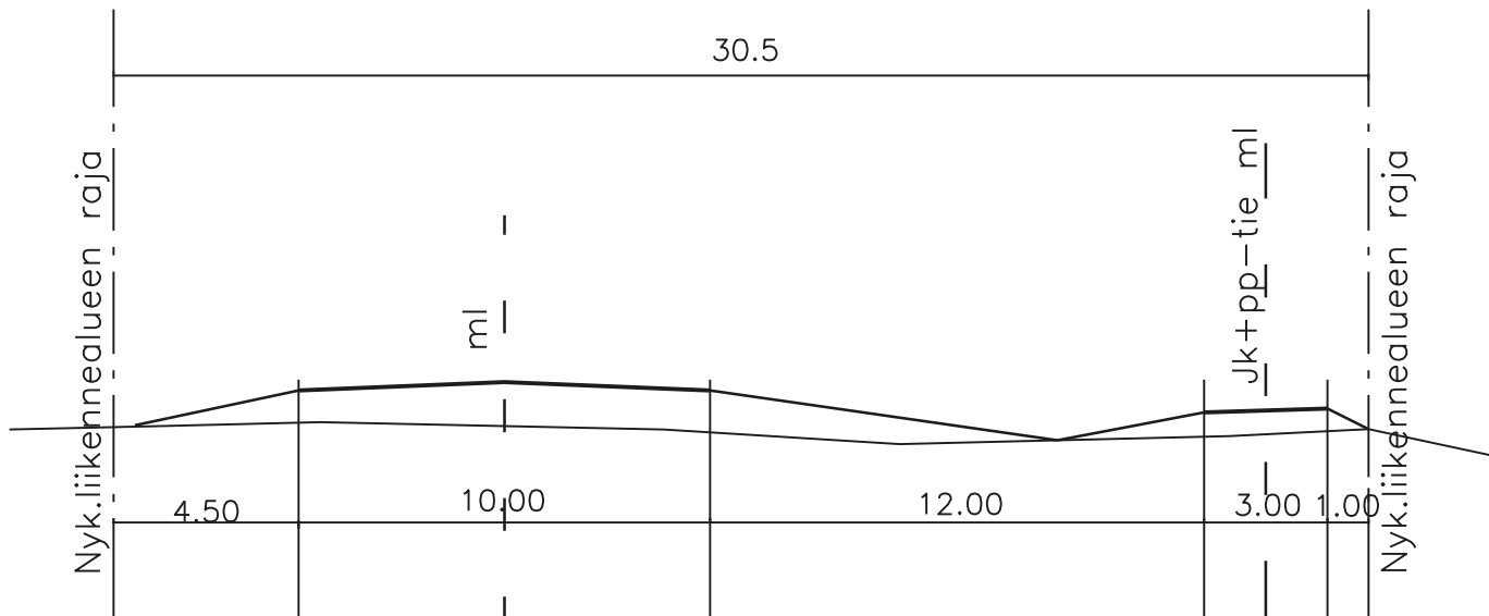
Laukaantien poikkileikkaus, nykytilanne
