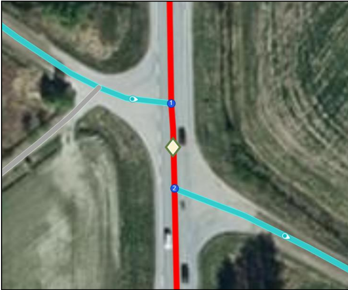
Kuva 27: Porrastettu liittymä
