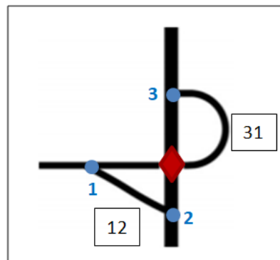
Kuva 10: Ramppien numerointi yksiramppisessa eritasoliittymässä
