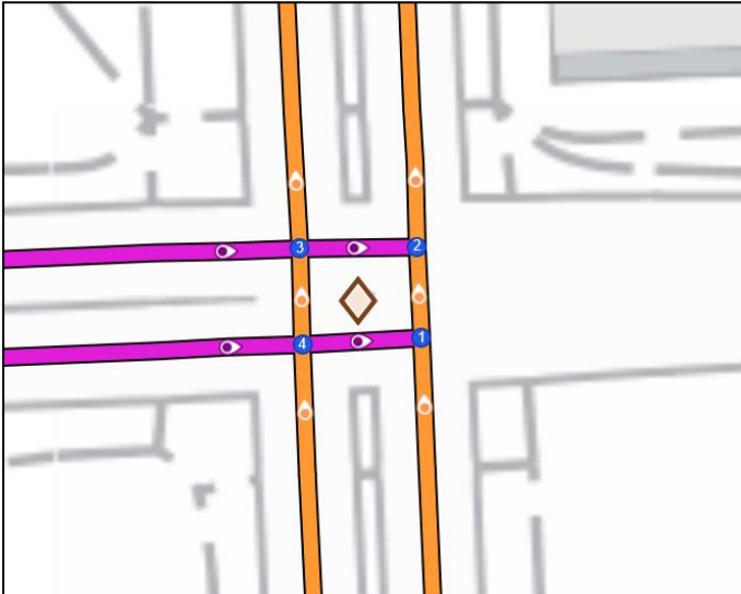
Kuva 18: Moniajoratainen liittymä: solmun sijainti ja liittymien numerointi
