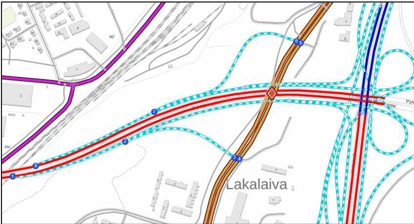
Kuva 17. Solmuun liitetään vain ne rampit ja liittymät joiden kautta on kulku ko. risteävälle tielle
