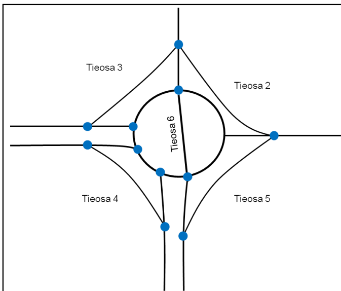
Kuva 12: Vapaille oikeille annetaan sama tienumero kuin kiertoliittymälle ja vastapäivään kasvava tieosnumero 2 - 5. Läpiajettavien kiertoliittymien läpiajolinjaus saa saman tienumeron kuin kiertoliittymä ja tieosnumeron 6 (vapaille oikeille jätetään tieosanumerovaraus, vaikka niitä ei olisikaan rakennettu)
