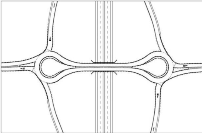
Kuva 11: Pisaraliittymät ramppien päissä. Kuva Väyläviraston julkaisusta Perusverkon eritasoliittymät Suunnitteluohje (Liikenneviraston ohjeita 39/2015)
