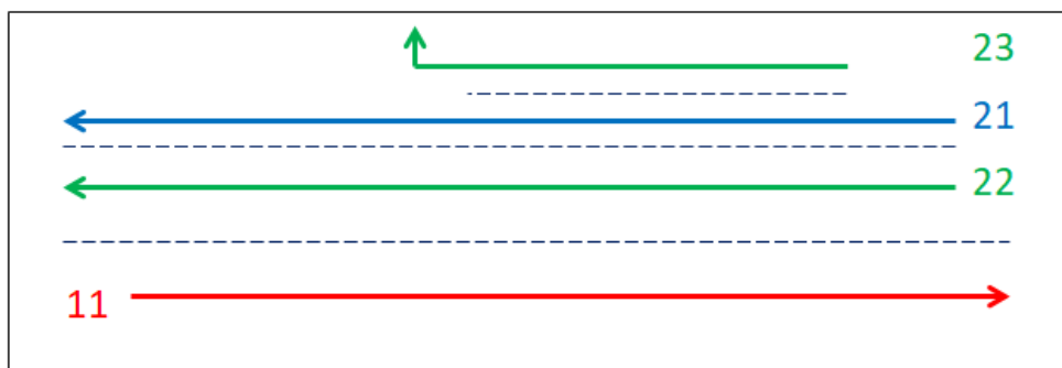
Kuva 11. Kääntymiskaista oikealle, kun ajosuunnassa 2 on myös ohituskaista
