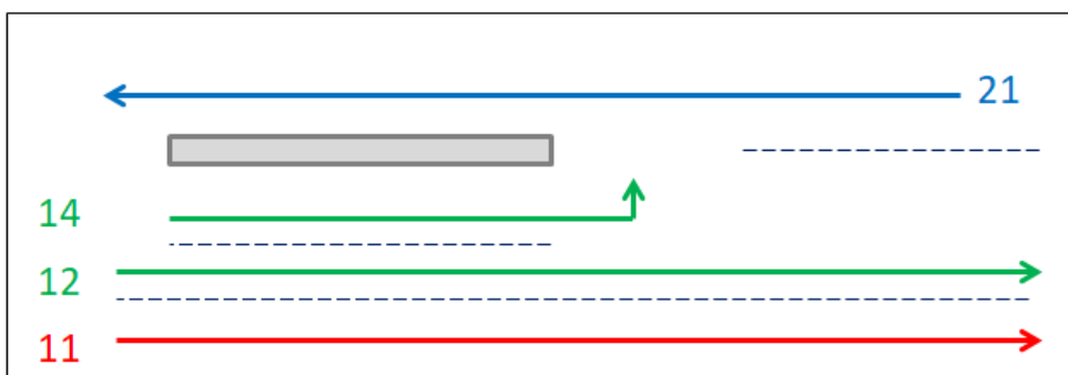
Kuva 8. Kääntymiskaista vasemmalle, kun ajosuunnassa 1 on myös ohituskaista
