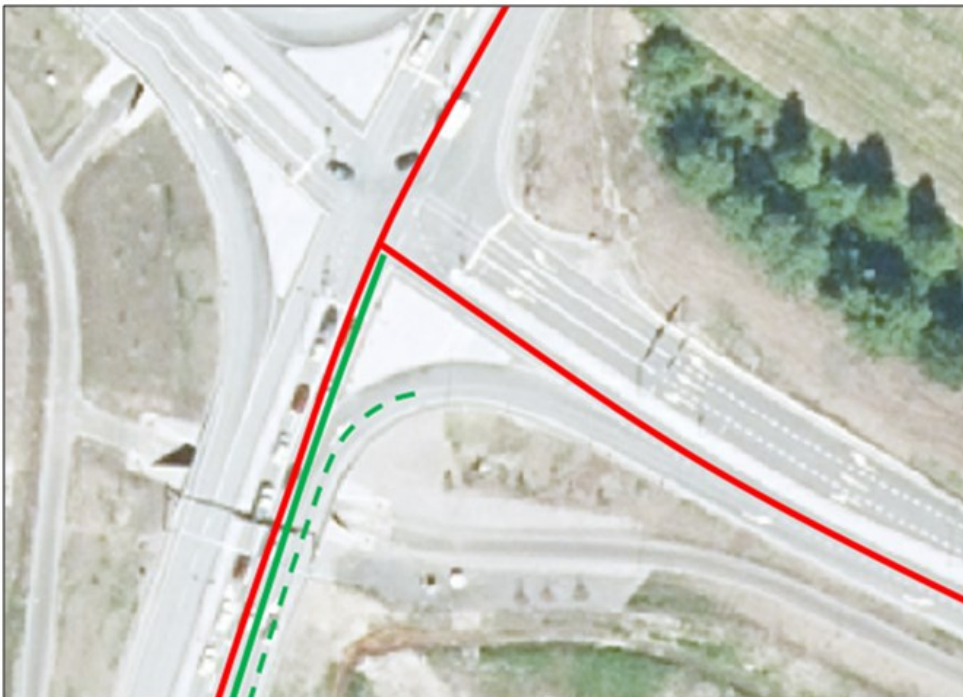
Kuva 18. Erkanemiskaista (vihreä) luodaan liittyvän tien risteykseen saakka. Todellinen linjaus on osoitettu katkoviivalla
