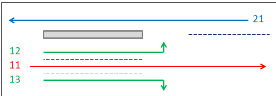
Kuva 5. Kääntymiskaistat liittymässä ajosuunnassa 1, ei ohituskaistoja
