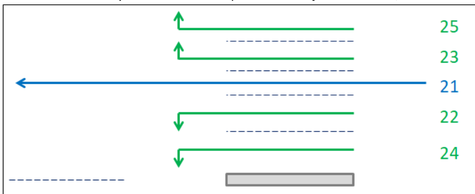
Kuva 15. Kaksi kääntymiskaistaa molempiin suuntiin ajosuunnassa 1, ei ohituskaistoja
