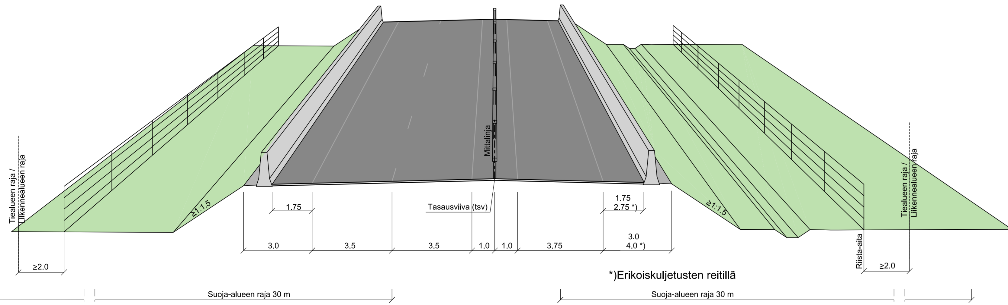
MELUVALLI / MELUAITA
