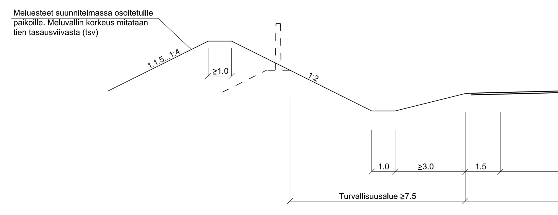
MELUVALLI / MELUAITA
