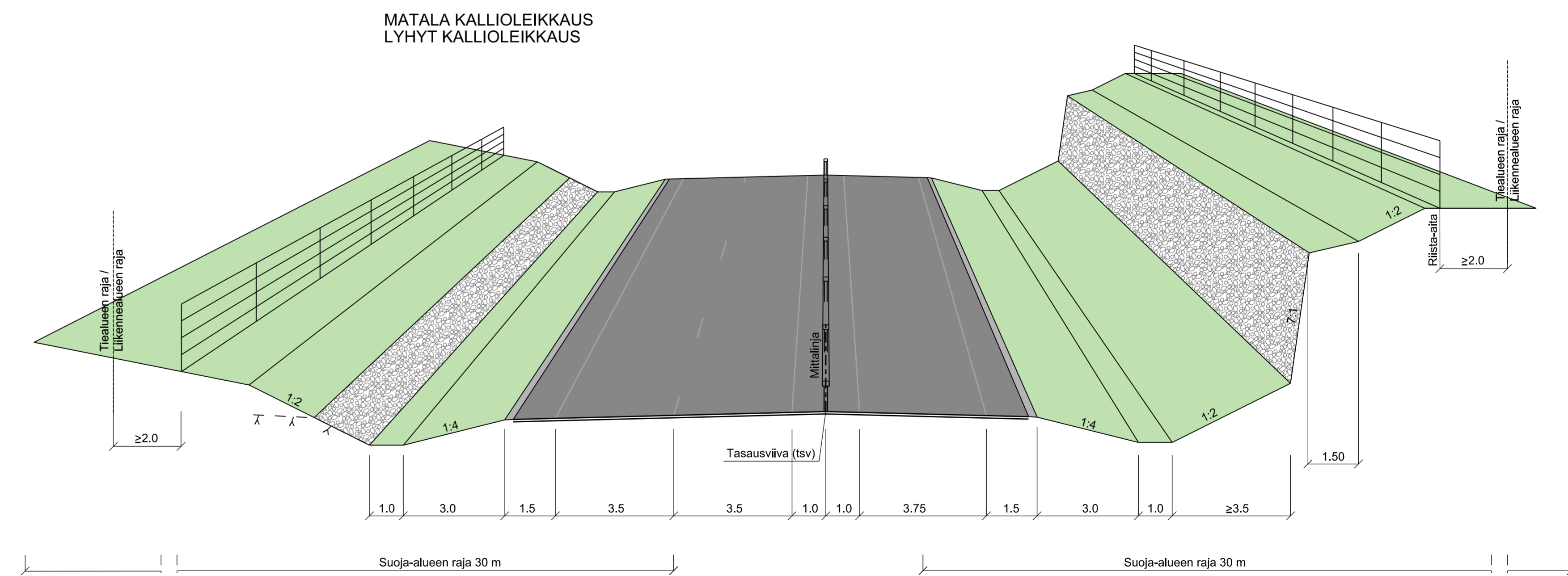
KORKEA KALLIOLEIKKAUS
