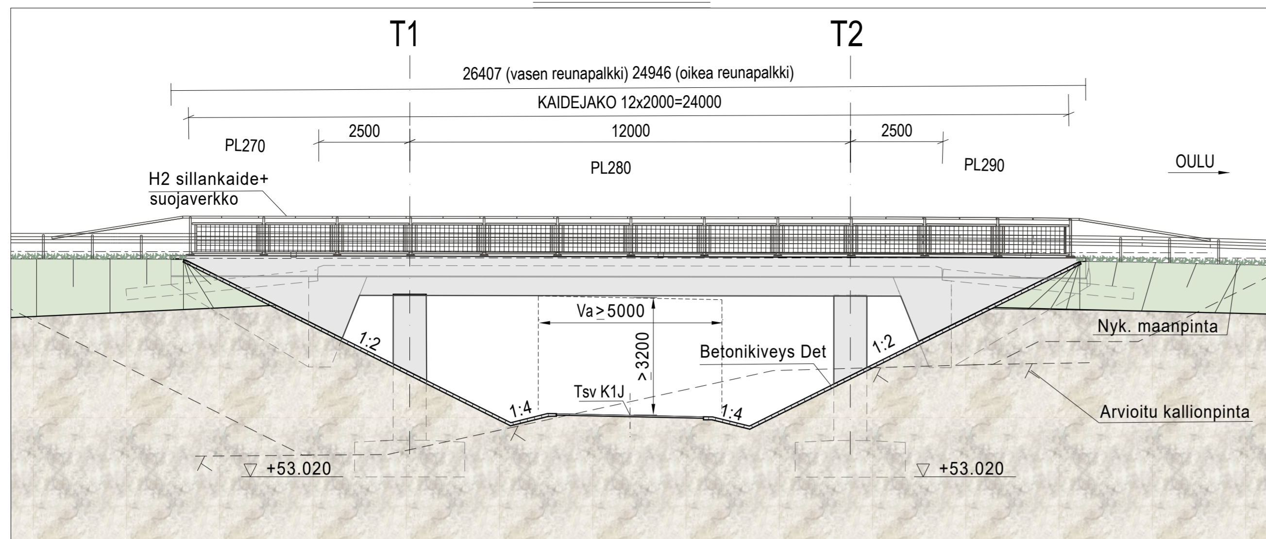
A-A 1:100
