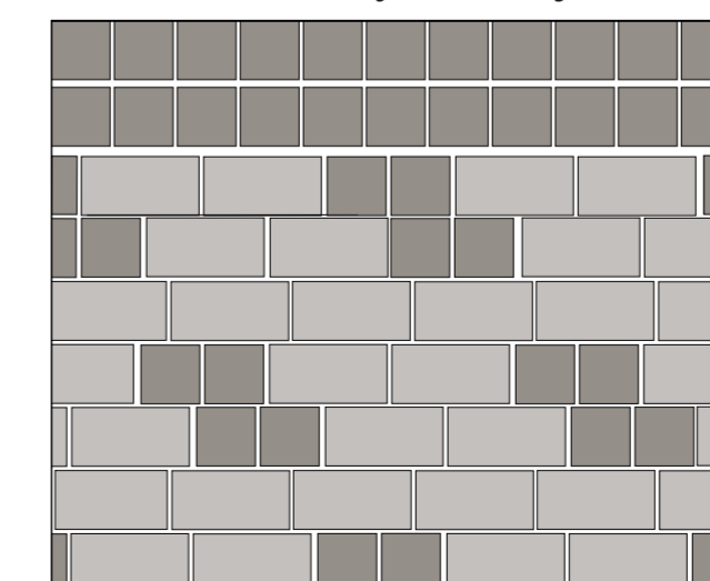
DET S1 kiveysdetalji 1:20
