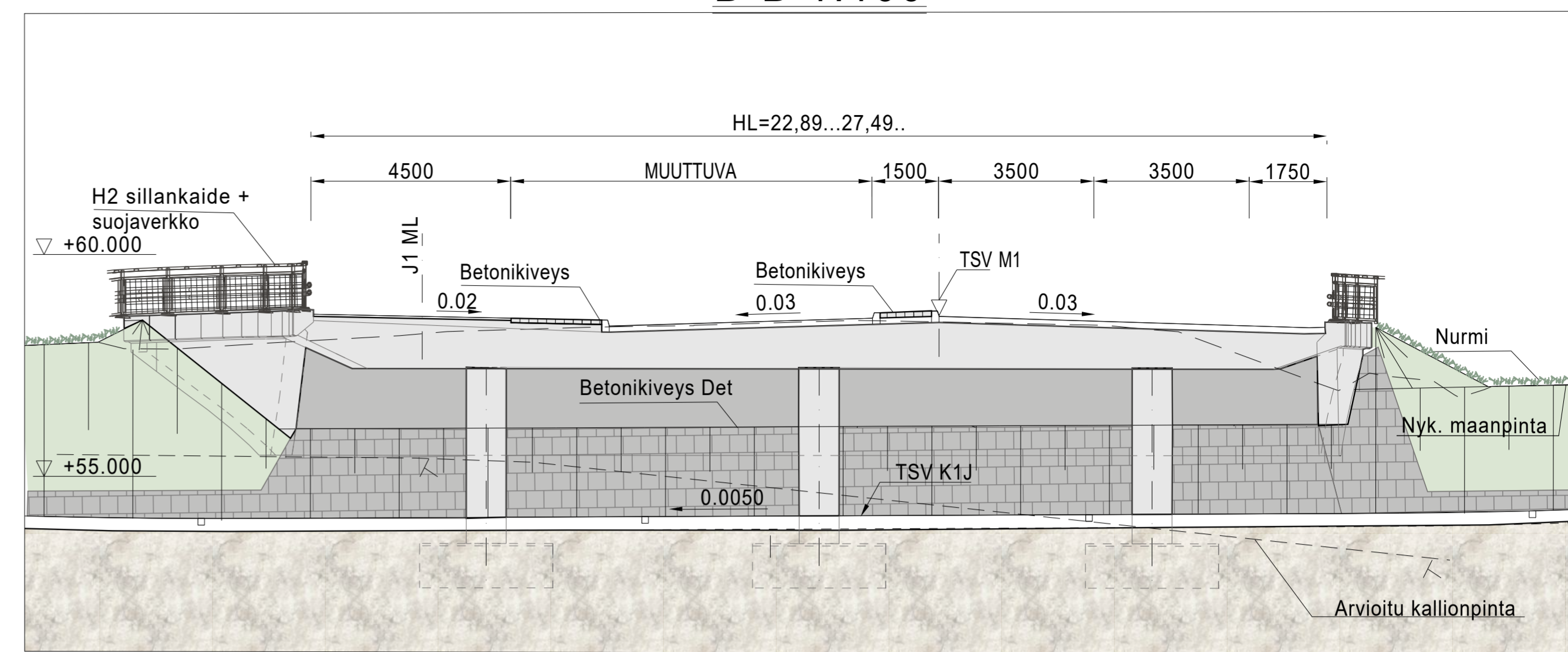
B-B 1:100
