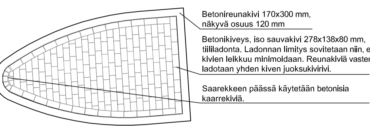
DETALJI 1 SAAREKKEIDEN LADONTA 1:20
