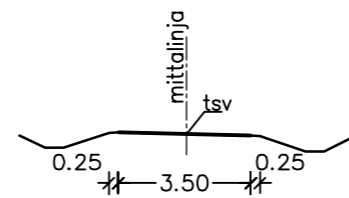
Peruspoikkileikkaus plv. 1-164
