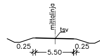
Peruspoikkileikkaus plv. 164-313
