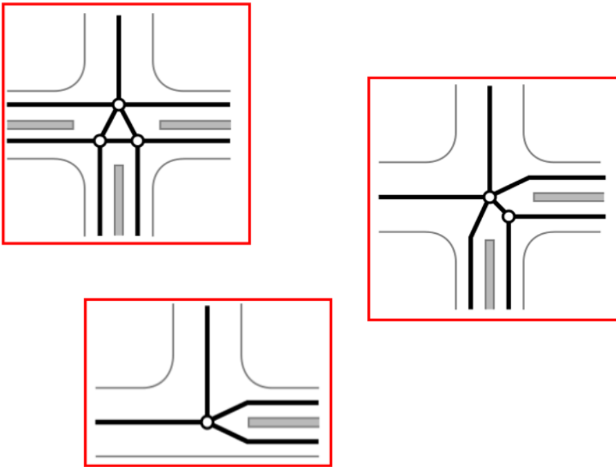
Kuva 31. Yleisimpien liittymätyyppien ratkaisumallit
