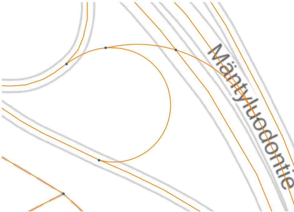
Kuva 45. Ainoastaan erikoiskuljetuksen käyttöön suunnitellut rampit mallinnetaan mukaan SURAVAGE aineistoon.
