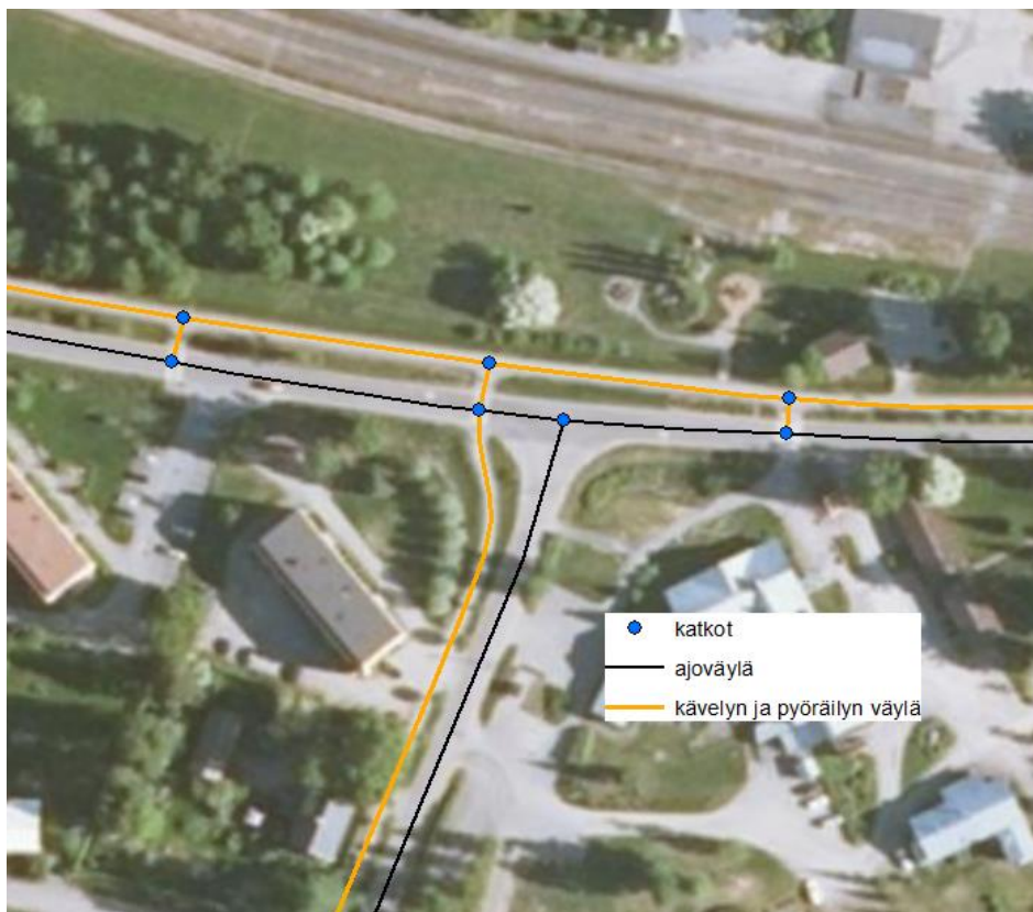
Kuva 9. Suojatien yhtymäkohdat tonteille tai pihoihin piirretään myös omana geometriana, mikäli kulkuyhteys erottuu erillisenä haarana.
