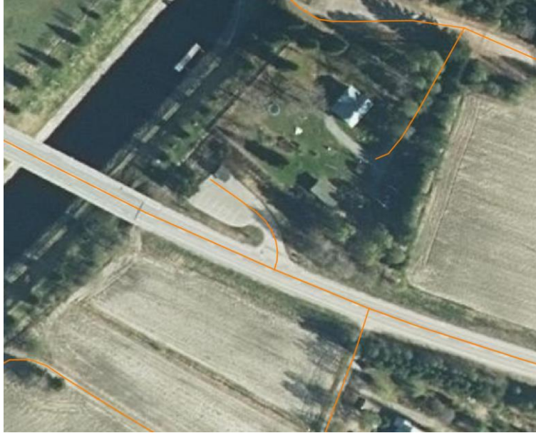
Kuva 38. Pussimallin levähdysalueella viiva viedään alueen päähän saakka.
