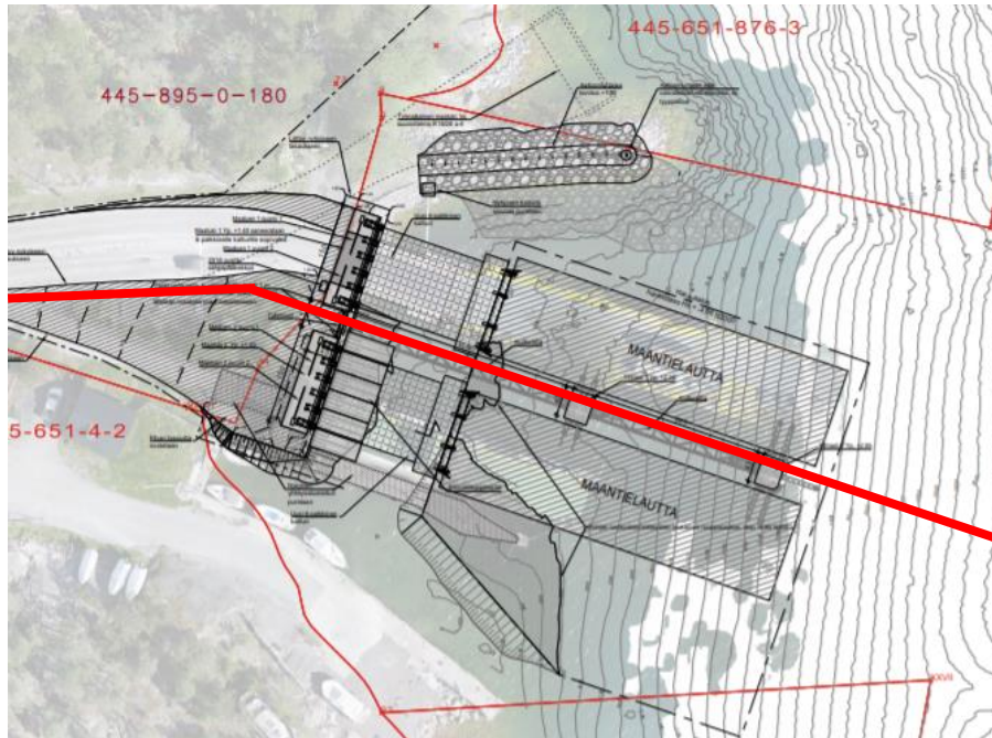
Kuva 42. Tuplalaiturirakenne, jolle johtaa yksi yhteinen tie. Tie tallennetaan yh- dellä keskilinjageometrialla, joka jatkuu tuplalaiturien keskilinjän mukaan lautta- väylänä merelle.
