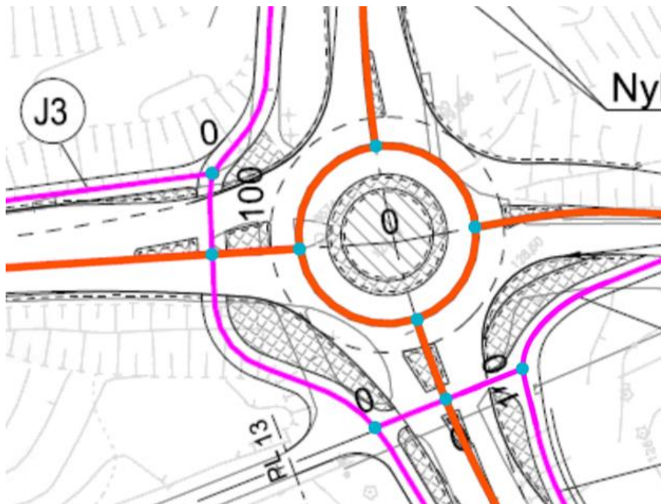
Kuva 22. Kiertoliittymästä kuvataan ajoradan keskilinjän säde. Kiertoliittymän keskilinja kuvataan myös murtoviivana.
