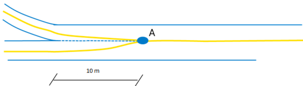
Kuva 13. Katkoskohtien muodostaminen tapauksessa, joissa liittymis- tai erkanemiskaista jatkuu omna kaistanaan tai jos ramppi erkanee pääväylän kääntymiskaistasta, muodostuu rampin geometria 10 metrin päähän rampin nokasta. Kuvan tapaus koskee molempia suuntia.
