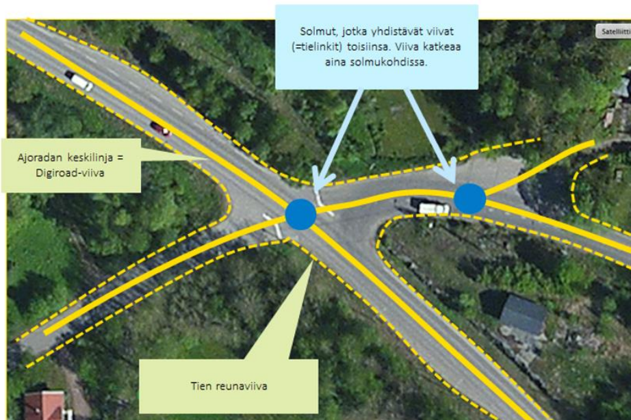
Kuva 46. Viivojen tulee katketa sinisellä merkityissä solmukohdissa. Katkeamiskohdissa viivojen päiden tulee liittyä toisiinsa saumattomasti ja ilman rakoa. Solmujen luonti on VVH-ylläpitäjän tehtävä, eli suunnittelijan ei tarvitse luoda solmuja.
