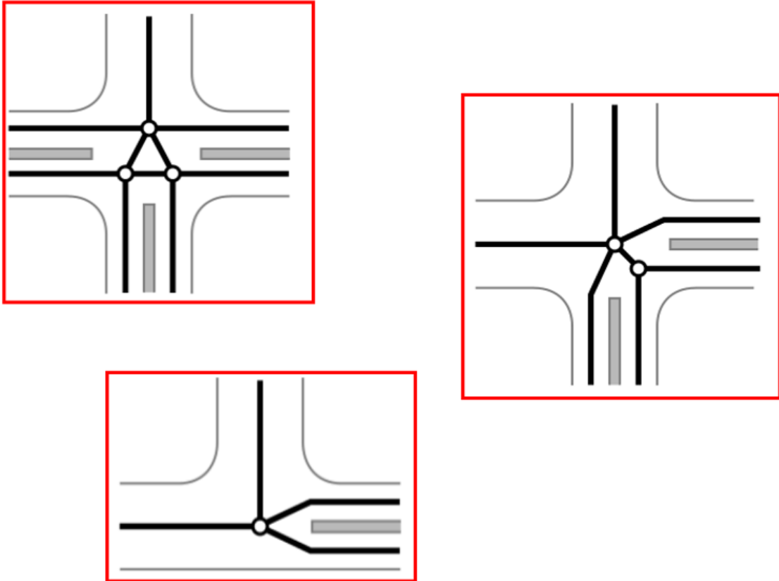
Kuva 31. Yleisimpien liittymätyyppien ratkaisumallit
