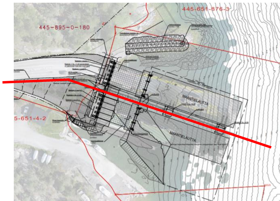
Kuva 42. Tuplalaiturirakenne, jolle johtaa yksi yhteinen tie. Tie tallennetaan yhdellä keskilinjageometrialla, joka jatkuu tuplalaiturien keskilinjän mukaan lauttaväylänä merelle.
