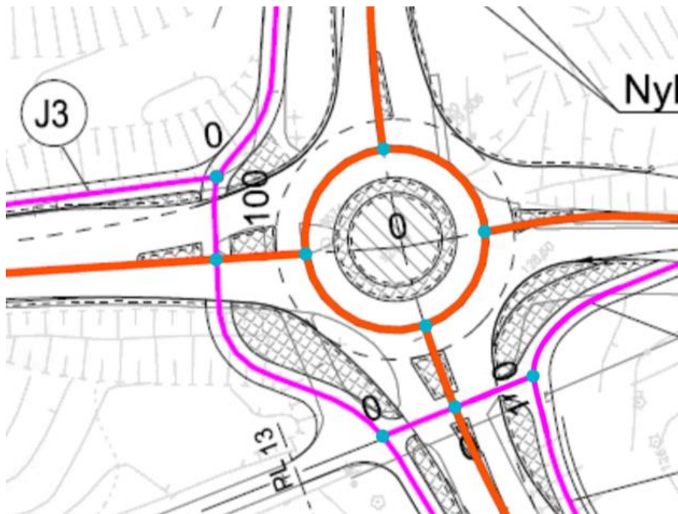
Kuva 22. Kiertoliittymästä kuvataan ajoradan keskilinjän säde. Kiertoliittymän keskilinja kuvataan myös murtoviivana.
