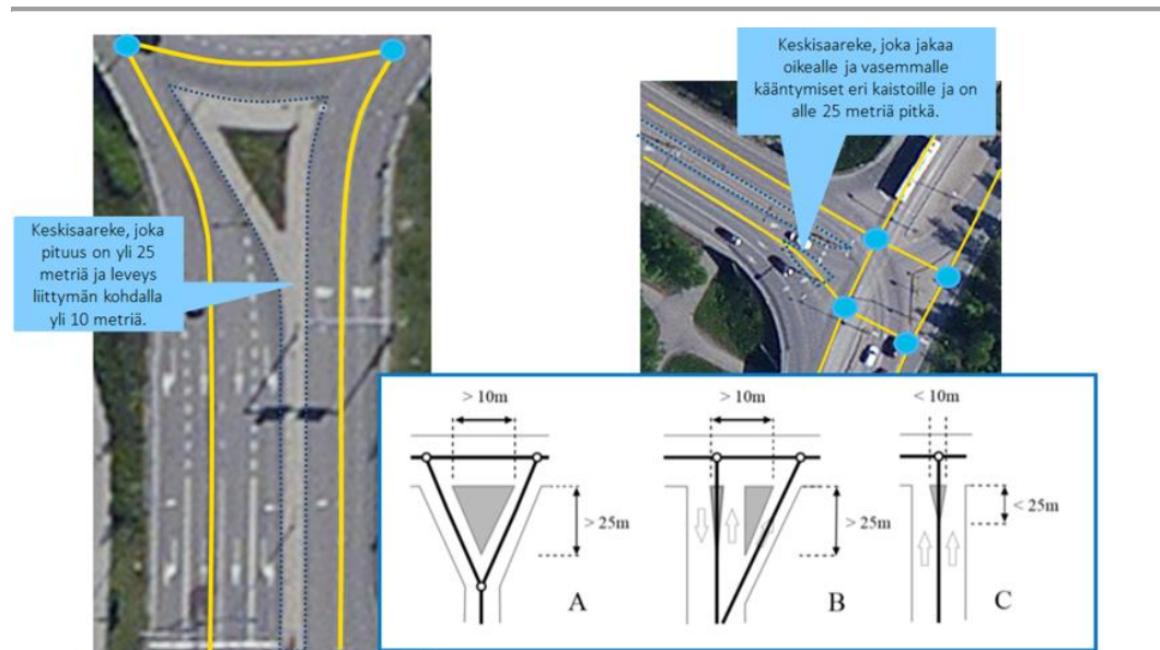
Kuva 29: Esimerkki haaraumien (ajoratojen jakautuminen) käsittelystä. Sekä pituus- että leveysehtojen tulee täyttyä.
