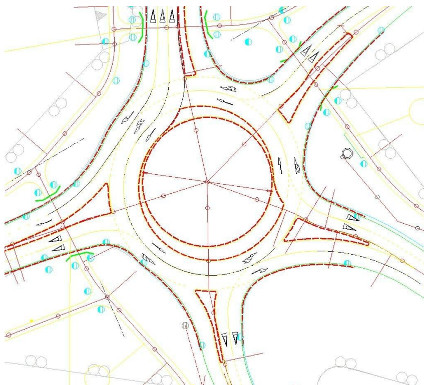
Kuva 8. Kiertoliittymä ja liikenteenjakajat dwg -tiedostossa. Ohut keltainen viiva kuvaa tien keskilinjaa, mutta se ei päde liikenneympyrässä ja liittymissä. Katkoviivalla on nähtävissä liikenteenjakajan ja kiertoliittymän polygonit, joita voi hyödyntää keskilinjan määrittämisessä QGIS:ssä.
