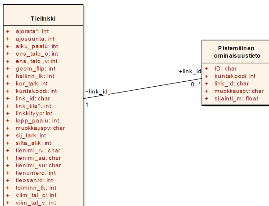
Bild 7: Punktformiga egenskapsuppgifter kan anknytas till väglänkar med hjälp av linjärreferering av länkens ID-egenskapsuppgift och m-värden.
