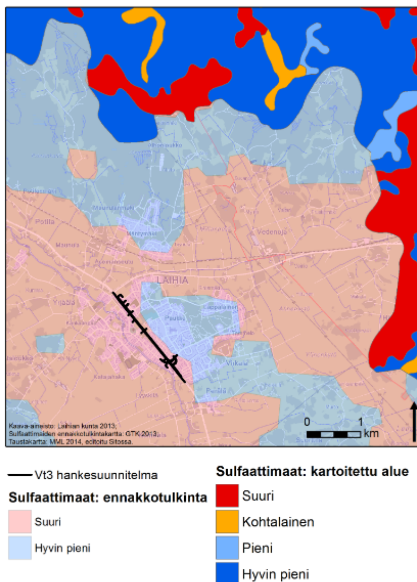
Kuva 10. Sulfaattimaiden ennakkotulkintakartta hankealueella ja sen läheisyydessä sekä lähimmät tutkitut alueet.
