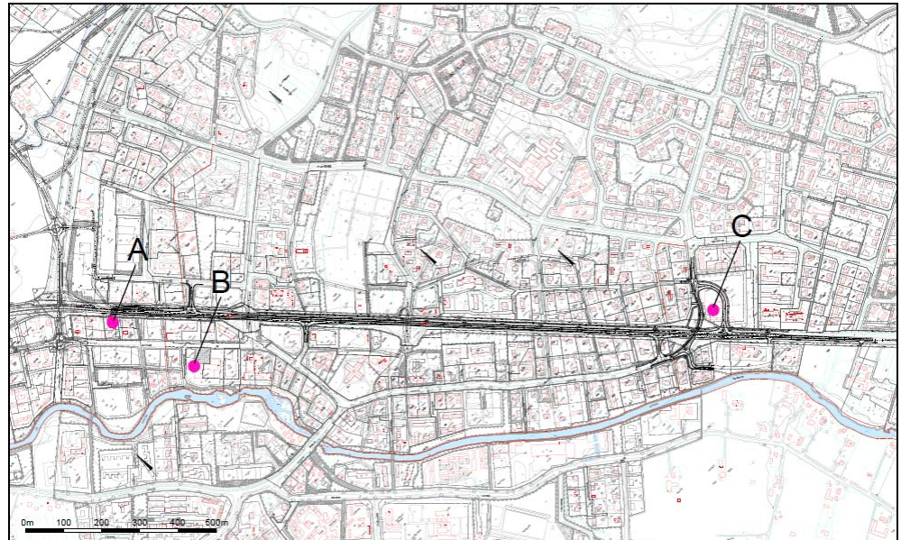
Kuva 9. Mahdolliset pilaantuneen maan kohteet.
