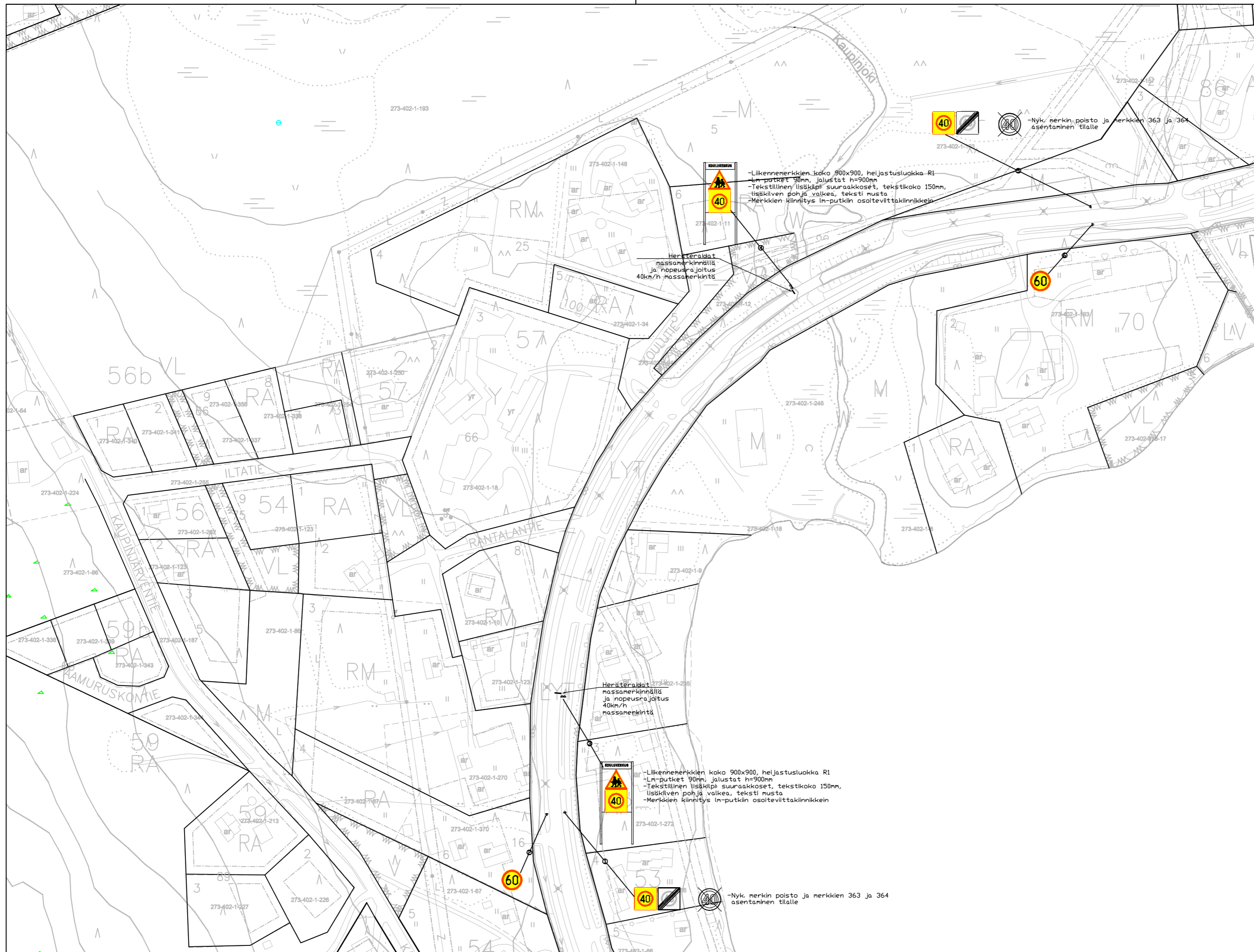
Mt940 Tiurajärventien liikenneturvallisuuden parantaminen Äkäslompolon koulun kohdalla LUONNOS 30.1.2019/Ramboll Finland Oy, TVAA
