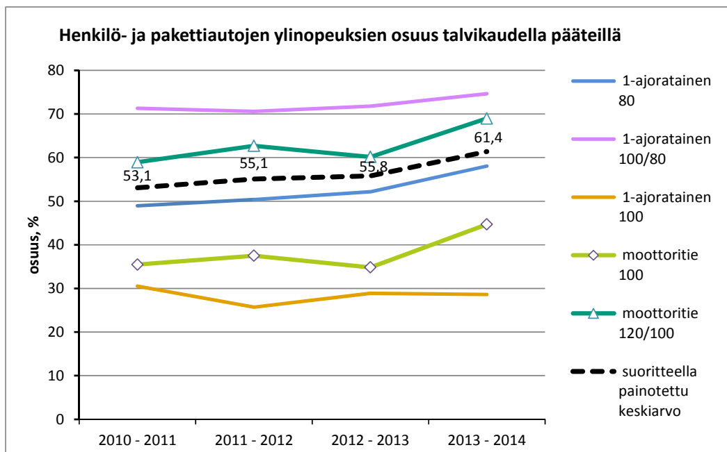
Kuva 13. Ylinopeutta ajavien henkilö- ja pakettiautojen osuus (%) tärkeimmissä tierryhmissä talvikausina 2011/2012–2013/2014.
