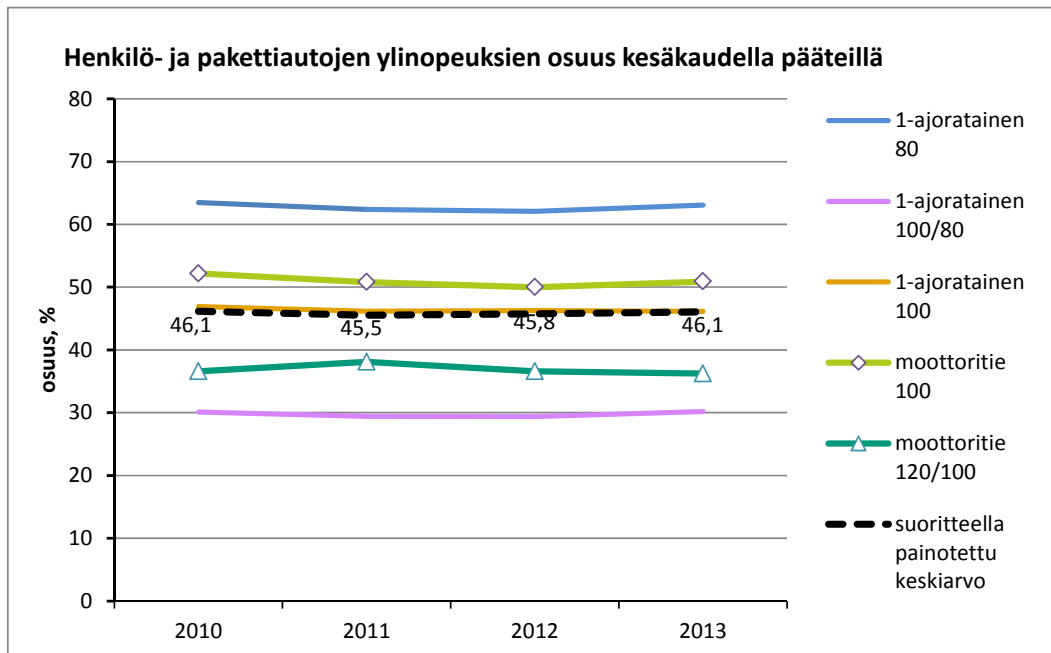
Kuva 7. Ylinopeutta ajavien henkilö- ja pakettiautojen osuus (%) tärkeimmissä tieryhmissä kesäkaudella vuosina 2010–2013.
