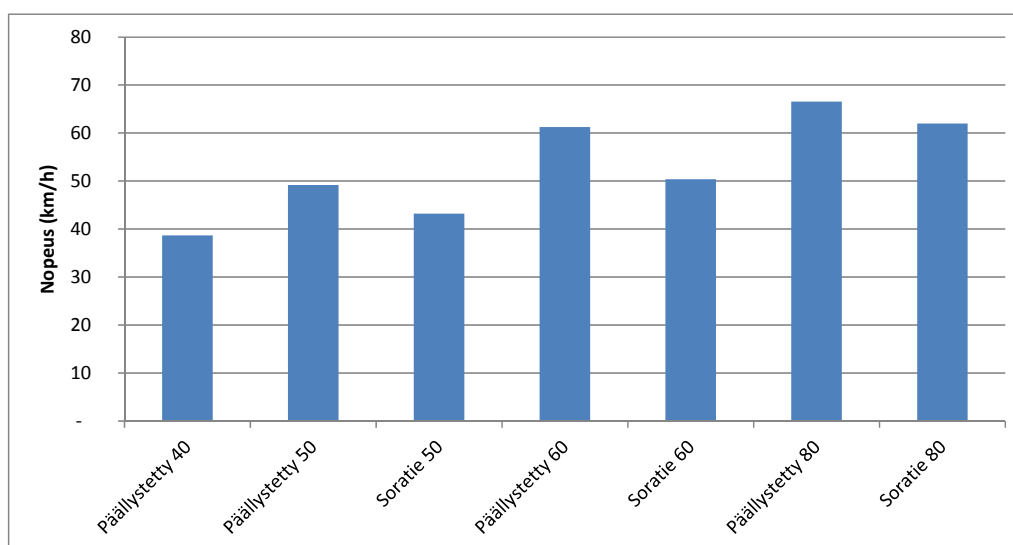
Kuva 15. Autoliikenteen keskinopeus alemman tieverkon teillä talvikautena 2012/2013. Kuvaan on valittu talven 2012/2013 nopeudet, koska ne ovat vertailukelpoisia kesän 2013 nopeuksien kanssa.
